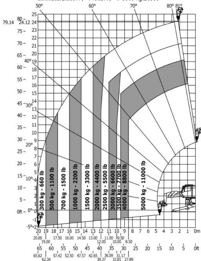
液压支腿完全打开，车身旋转，带 5000 kg 卷扬机
