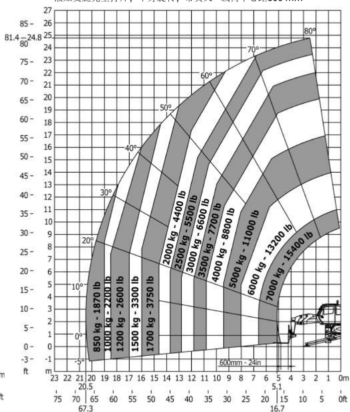
液压支腿完全打开, 车身旋转, 带货叉 - 载荷中心距600 mm
