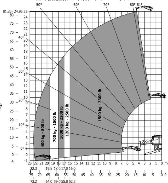
液压支腿完全打开，车身旋转，带 1500 kg 吊臂
