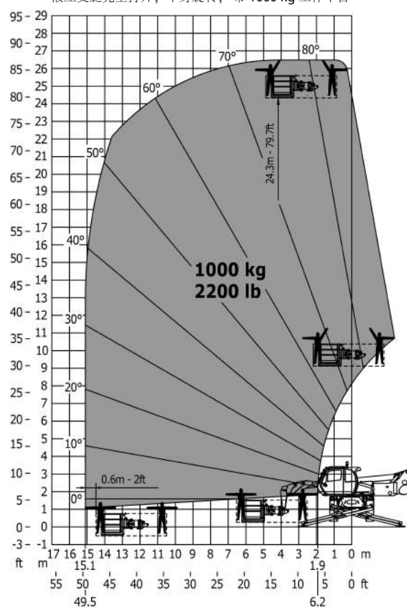
液压支腿完全打开，车身旋转，带 1000 kg 工作平台
