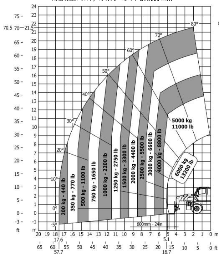
液压支腿未打开, 带货叉 - 载荷中心距600 mm
