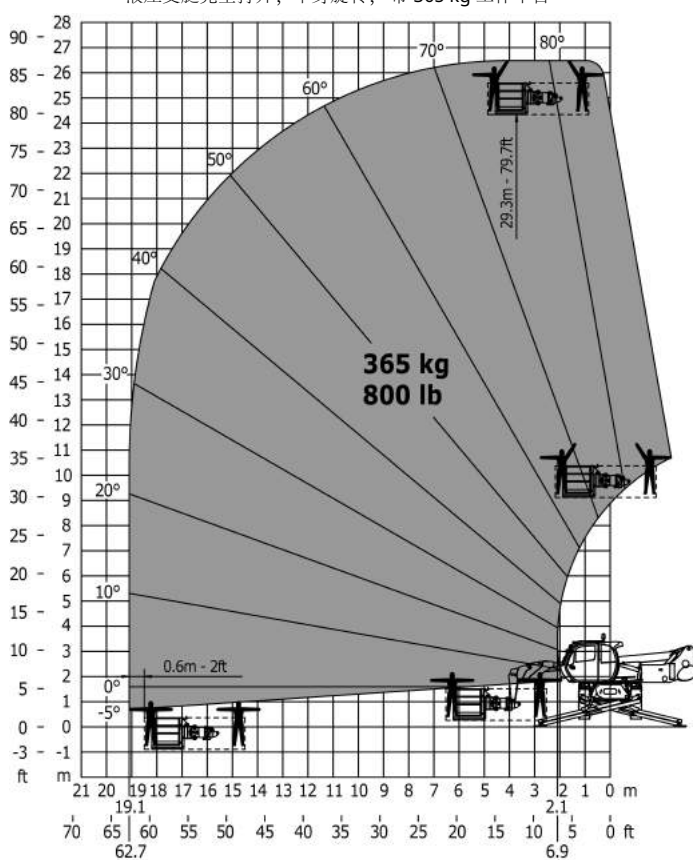
液压支腿完全打开，车身旋转，带 365 kg 工作平台
